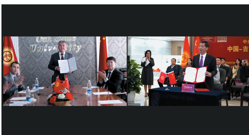
校党委副书记、校长郭广生通过视频方式与奥什国立大学校长阔杰别科夫签署两校学生交换协议。
